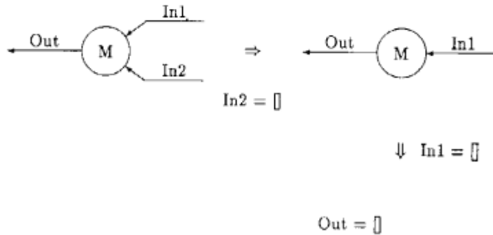
図 10.7: 組込みマージ (4)
