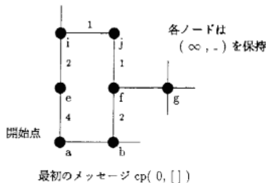
図 8.6: 最初のメッセージ
