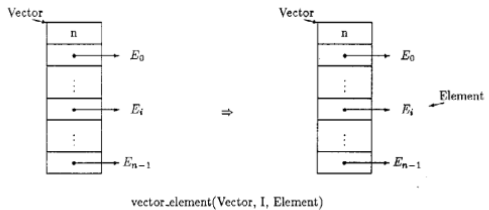
図 10.17: ベクタの要素の参照 (1)
