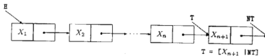
図 5.9: 差分リスト (H, NT)
