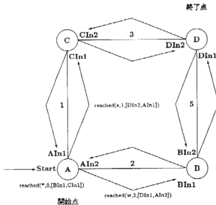
図 15.7: 実行開始直後の状態
