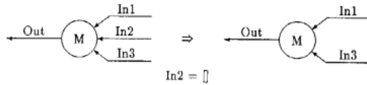
図 10.7: 組込みマージ (4)
