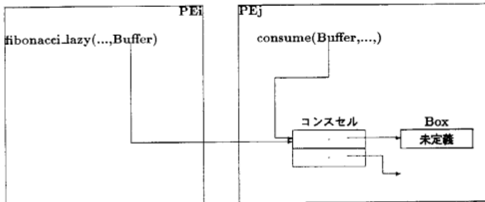
図 16.1: プロセッサ間における有限長バッファ (1)
