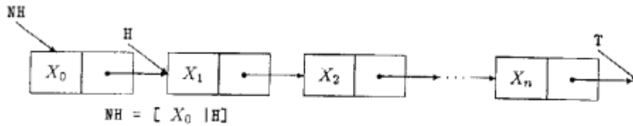
図 5.7: 差分リスト (NH, T)
