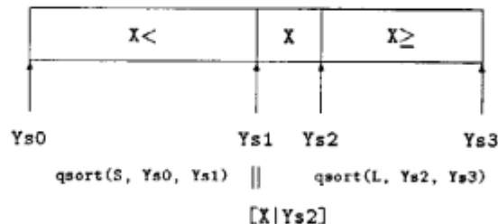
図 8.4: \text{qsort}(Xs, Ys0, Ys3) の結果の構成
