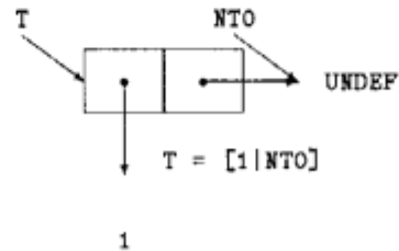
図 5.11: キューの状態 (1)
