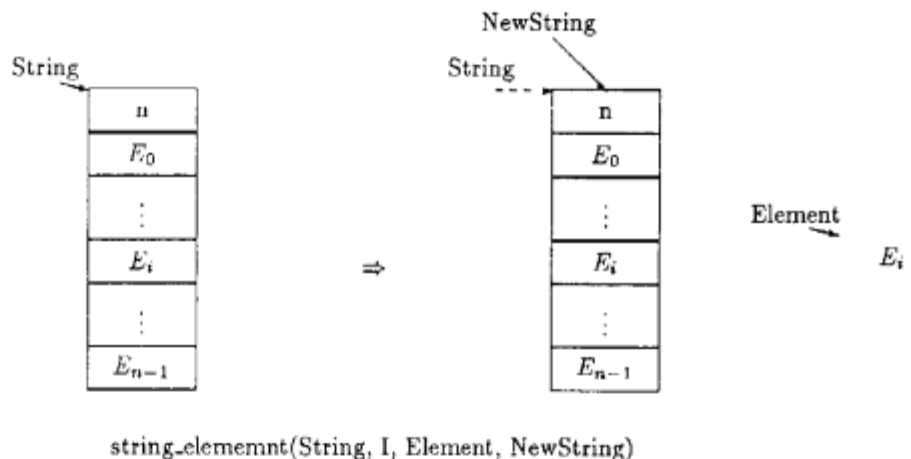
図 10.10: ストリングの要素の参照 (1)
