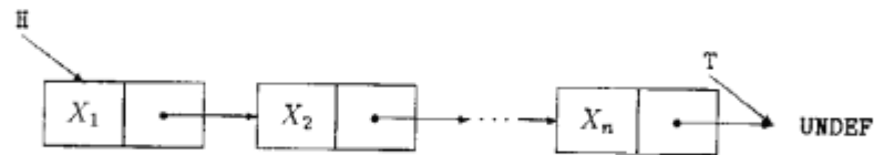
図 5.7: 差分リスト (NH, T)
