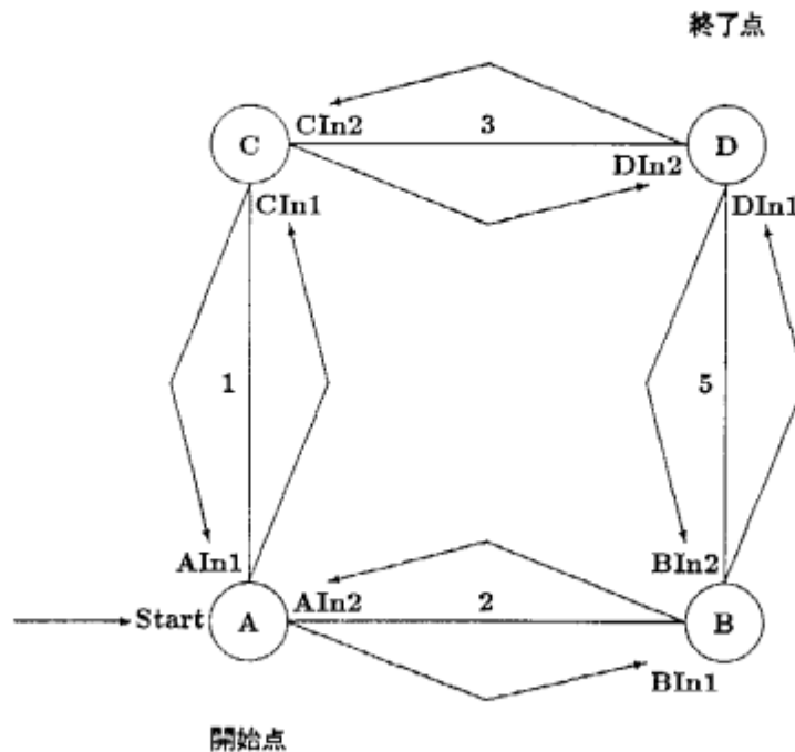
図 15.6: 最適経路問題のネットワーク (2)
