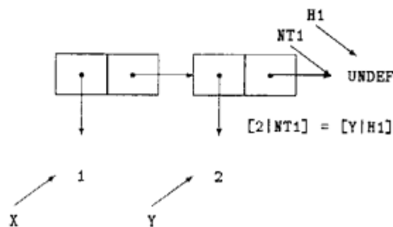
図 5.14: キューの状態 (4)
