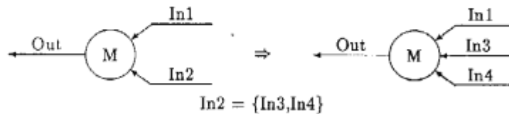
図 10.6: 組込みマージャ (3)
