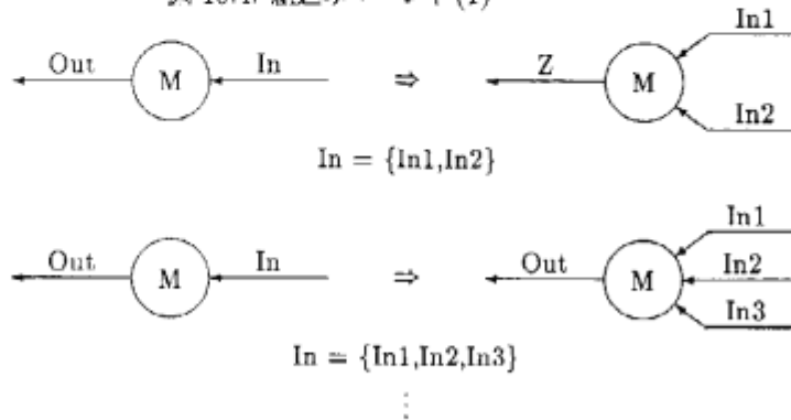
図 10.4: 組込みマージャ (1)
