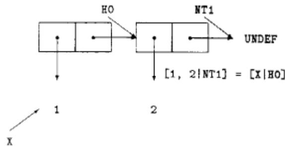
図 5.13: キューの状態 (3)
