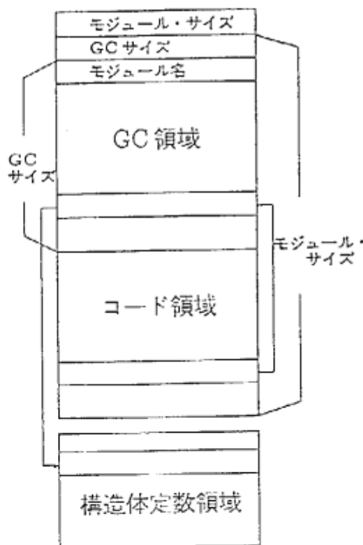
図1: モジュールの形式と構造体定数領域
