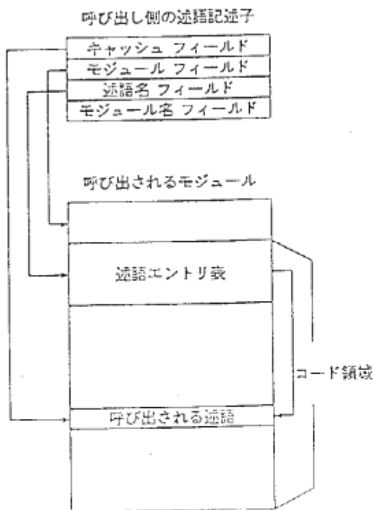
図 2: モジュール外呼び出し。
